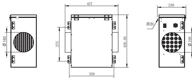
EFE尺寸图单位(mm)
